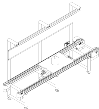
ZY01.C2: C型双层自由滚轮线
