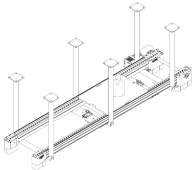
ZY01.B2: B型双层自由滚轮线
